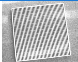
方形
