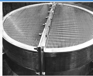
圆形
