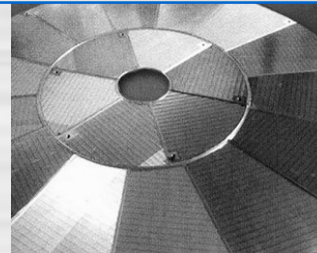
扇形
