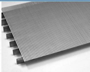
长方形
